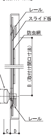
【縦断面図】
