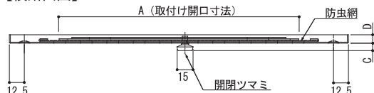
【外観図】
