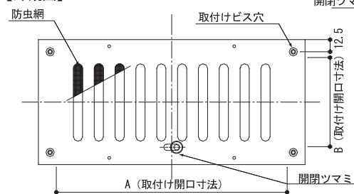
【外観図】
