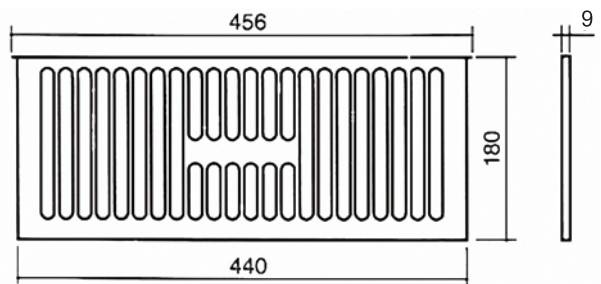
■仕様図 IMB-YS4418 / IMB-YSS4418
