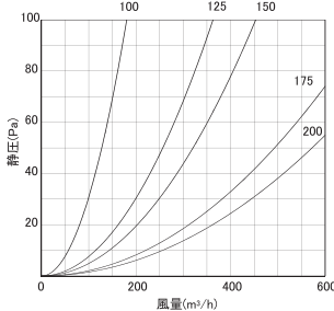
圧力損失特性
