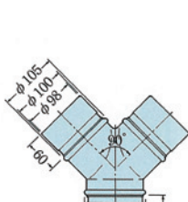
樹脂製分岐Y管
