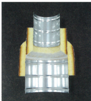
断面図
